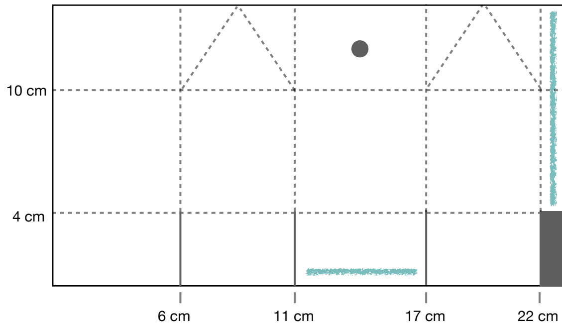
Farbkarton 15 cm x 23 cm
